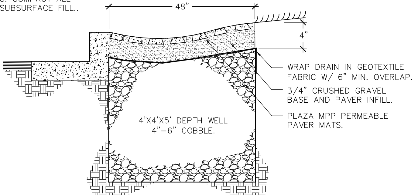
PERMEABLE PAVER EDGE GRAVEL SUMP
